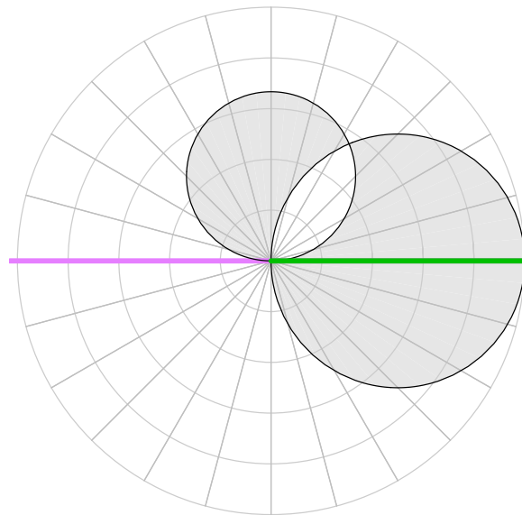
Fig. Polar coordinates
